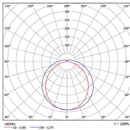
配光曲線
